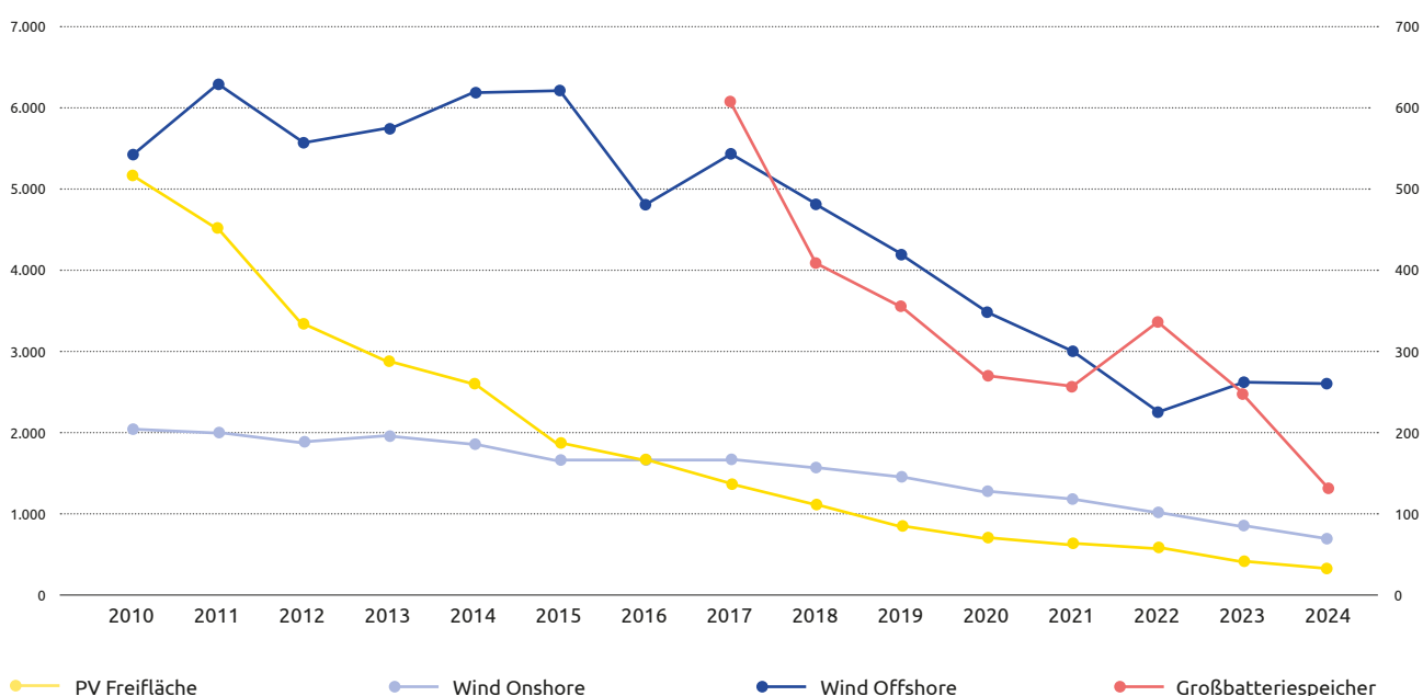
Kosten für Erneuerbare Energien & Großbatteriespeicher (in USD/kW; USD/kWh für Speicher)
