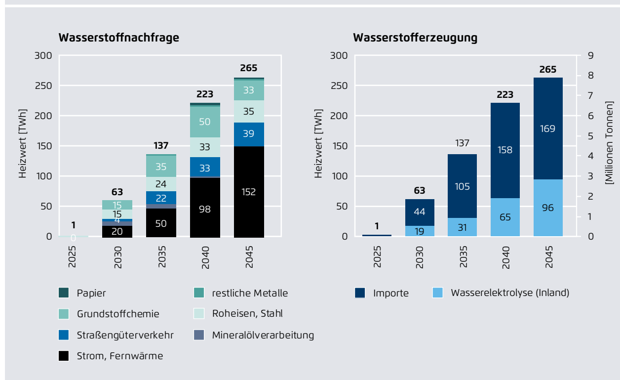
CO 2 -freie Wasserstofferzeugung und -nutzung in Deutschland
