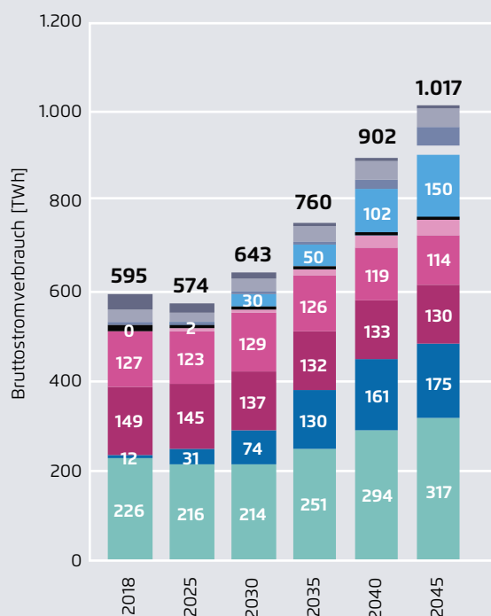
Bruttostromverbrauch
